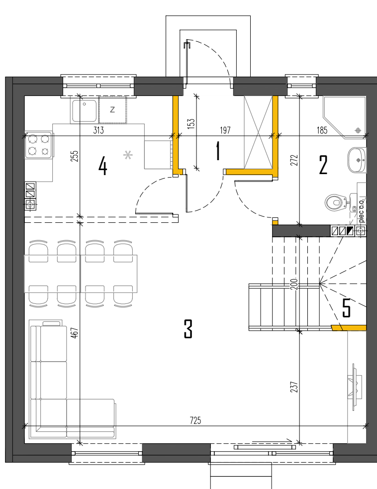
RZUT PARTERU
